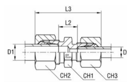
B3-vágógyűrűvel
