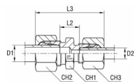
B3-vágógyűrűvel
