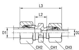
B4-vágógyűrűvel
