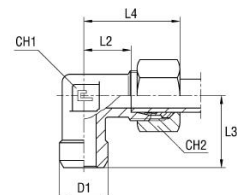
mit B3-Schneidring
