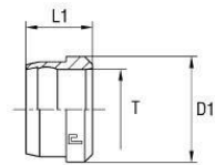
B3-řezný kroužek
