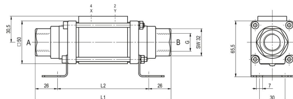
CVTE-10 Funkce NO
