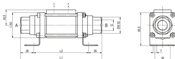
CVTE-10 Funkce NC
