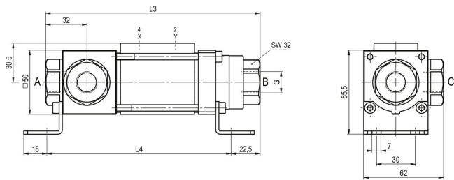
CVTE3-10 Funkce NO (> 63bar)
