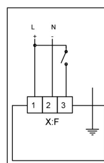
2-pontos vezérlés
