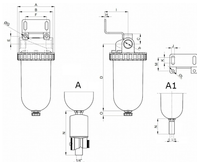
A, A1: avtomatski izpustni ventil
