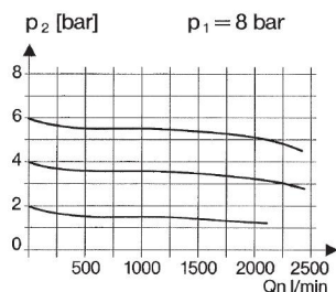
Átfolyási diagram
