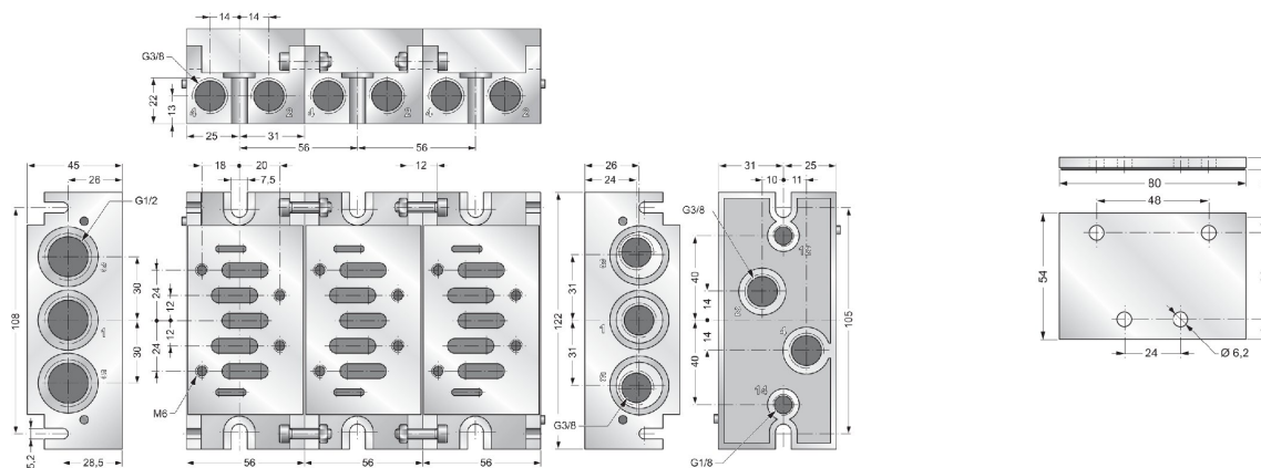
Připojovací díl Typ BT12
