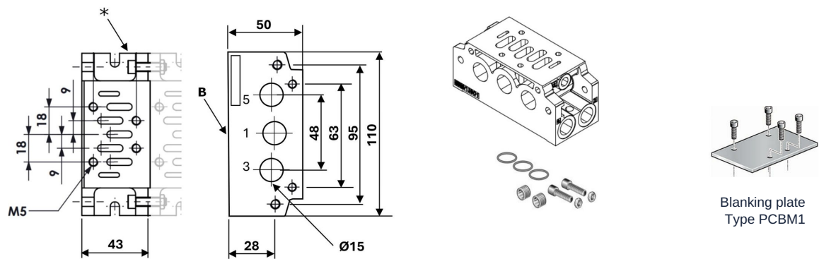
Center piece type SBI1-CE
