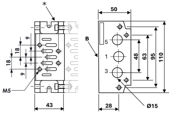
Element środkowy typ SBI1-CE
