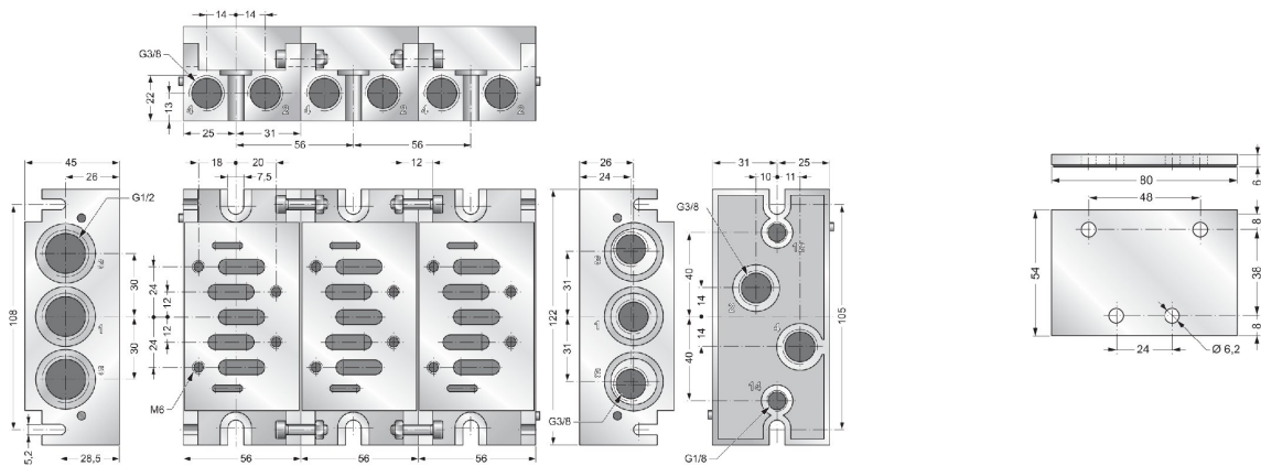
Središnji deo Typ BMI2
