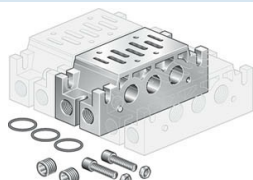
Središnji deo Typ BMI2
