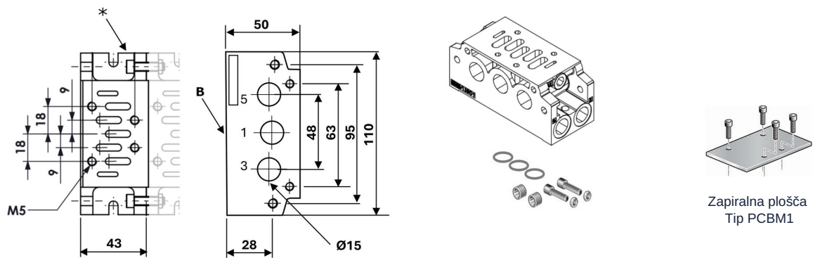
Srednji del tipa SBI1-CE
