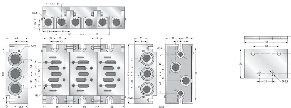
Priključni kos Typ BTI2
