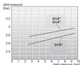
Acționare pneumatic/arcă
