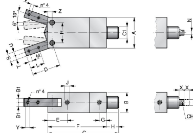
Versie doorlopende zuigerstang:
