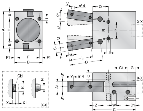
Versie doorlopende zuigerstang
