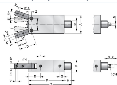
Version genomgående kolvstång:
