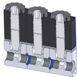
Montage der O-Ringe
