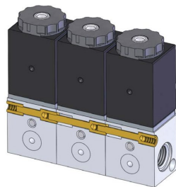
Montage der Verbindungsschrauben
