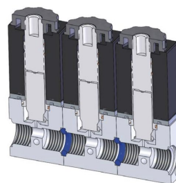
O-renkaiden asennus
