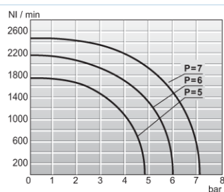
Virtauskaavio 1/4"
