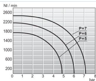
Virtauskaavio 1/4"
