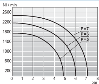
Flödesdiagramm 1/4"
