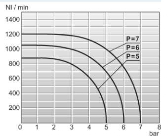
Flödesdiagramm 1/8"
