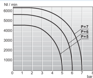
Flödesdiagramm 1/2"
