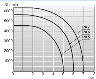
Diagramme de débit 1/2"
