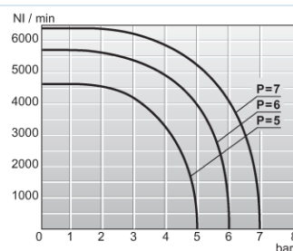
Διάγραμμα ροής 1/2"
