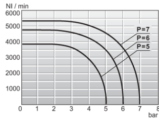
Diagrama de caudal 1/2"
