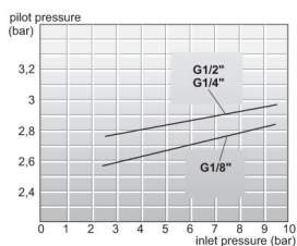
Aktivering pneumatisk/fjeder
