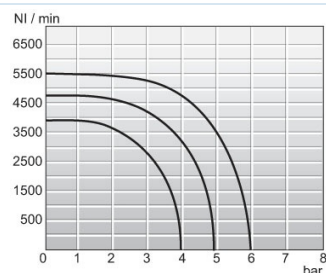
Virtauskaavio 1/2"
