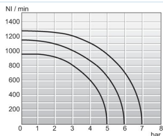
Virtauskaavio 1/8"
