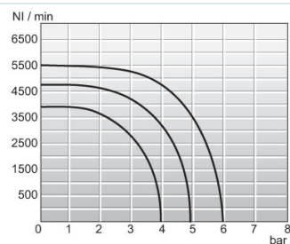
Doorstroomdiagramma 1/2"
