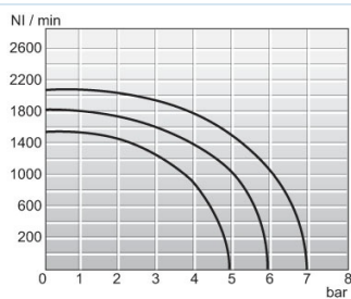
Doorstroomdiagramma 1/4"
