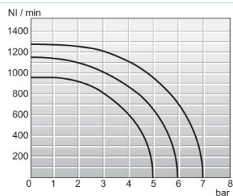
Doorstroomdiagramma 1/8"
