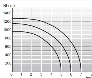
Διάγραμμα ροής 1/8"
