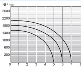
Διάγραμμα ροής 1/4"
