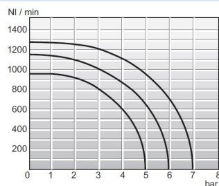
Virtauskaavio 1/8"
