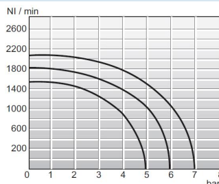
Virtauskaavio 1/4"
