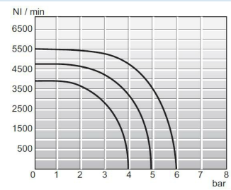
Virtauskaavio 1/2"
