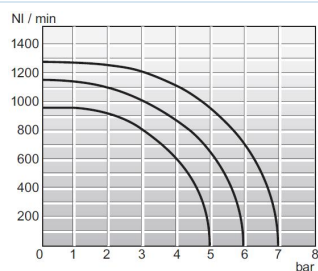
Strømningsdiagramm 1/8"
