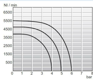
Strømningsdiagramm 1/2"
