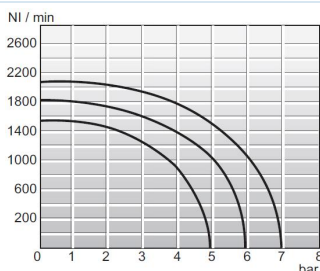
Strømningsdiagramm 1/4"
