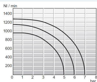
Doorstroomdiagramma 1/8"
