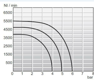
Διάγραμμα ροής 1/2"
