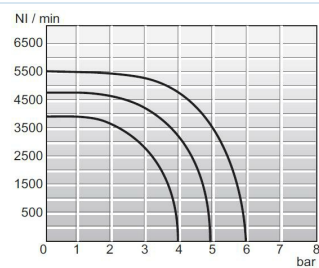
Doorstroombiagramma 1/2"
