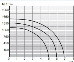
Virtauskaavio 1/4"
