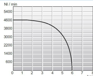
Virtauskaavio 1/2"
