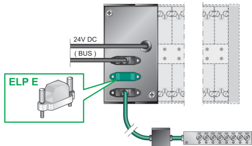
ELP I Connecteur de terminaison pour INPUT PORT
