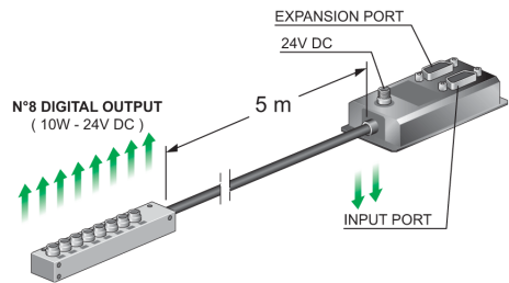
SCBO 88-M Boîtier pour 8 sorties numériques (10W - 24V DC)
