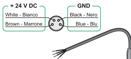
CW-PS Forsyningsspenningskabel
