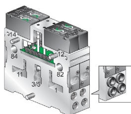
Modul pentru stație de electrovalve electric/electric - _ _ -
