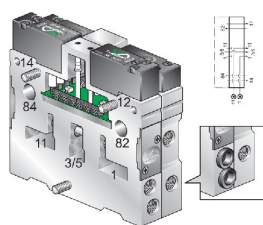
Modul Separator de presiune de lucru - _ Y - cu modul de stație individuală
