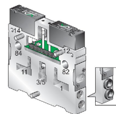
Modul cu stație individuală
