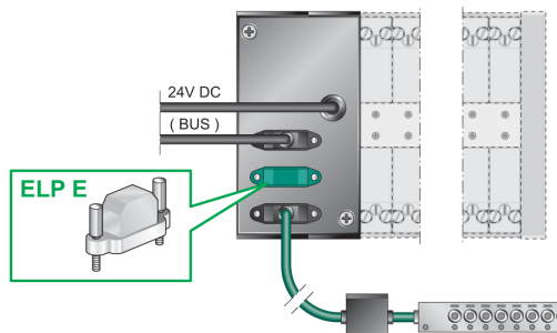
ELP I Ștecher de terminare pentru INPUT PORT
