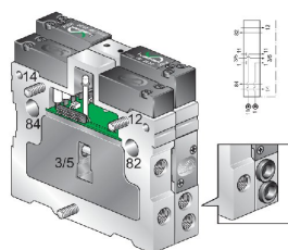
Modul Separator de presiune de lucru - X _ - cu modul de stație individuală
