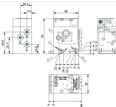
Σχέδιο διαστάσεων
