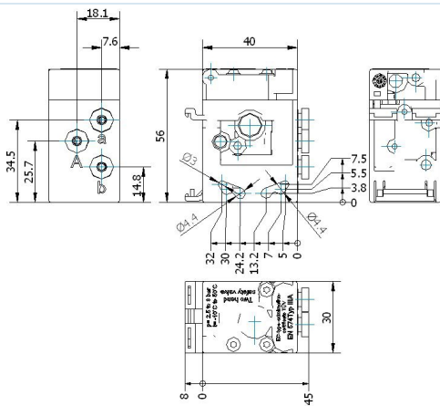
Plano acotado
