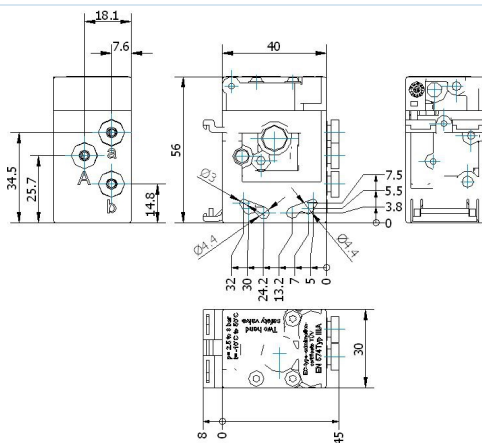
Méretrajz
