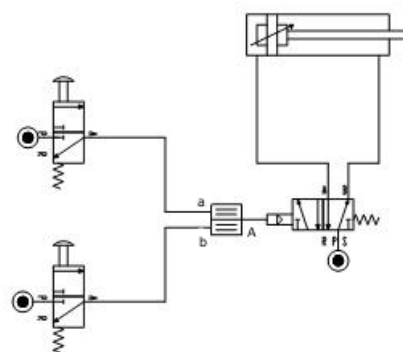
Tilkoblingsskisse
