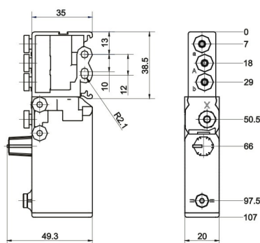
Dimenzijski crtež
