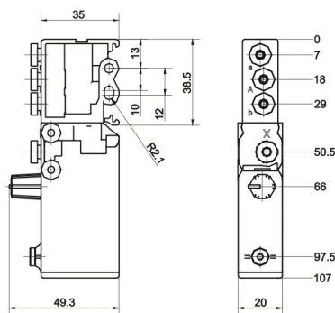
Disegno quotato
