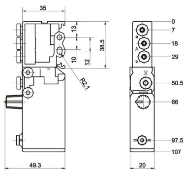
Disegno quotato
