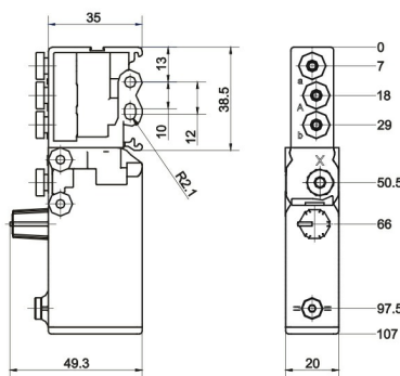
Desen dimensional
