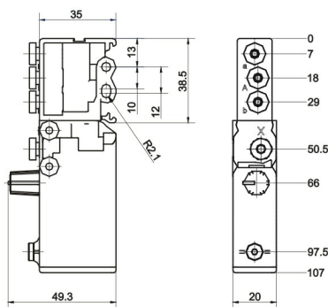
Dimenzioni crtež
