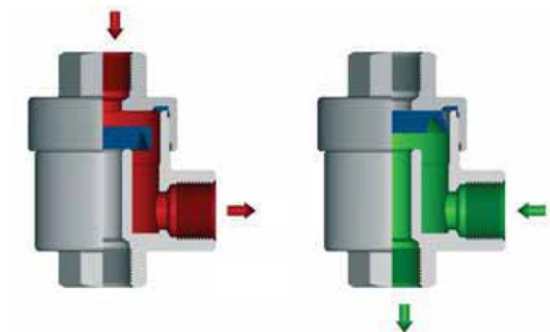
Strømningsretning til sylinder
