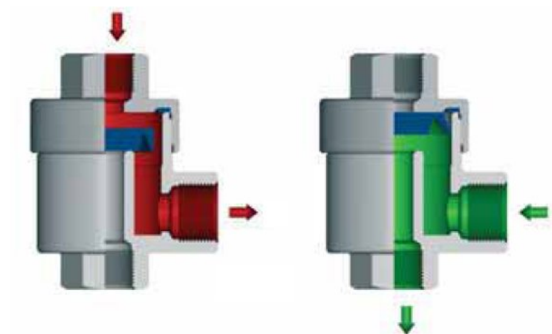
Flödesriktning till cylindern
