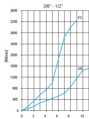
Omdreining på spindelen
