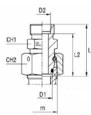
Grundkropp
